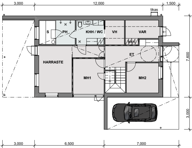
VAIHTOEHTOINEN POHJA, 1.KERROS
