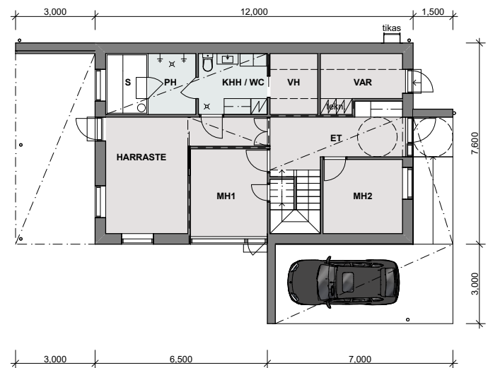
VAIHTOEHTOINEN POHJA, 1.KERROS
